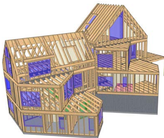
Konstruksjonstegning av Thaulowbakken 1.
