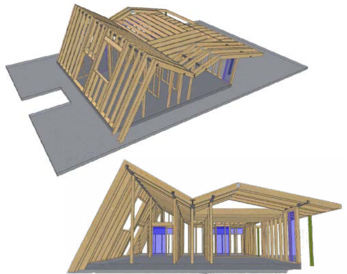
Konstruksjonstegning av Saunaen i Lofoten for DSN Entreprenør.
